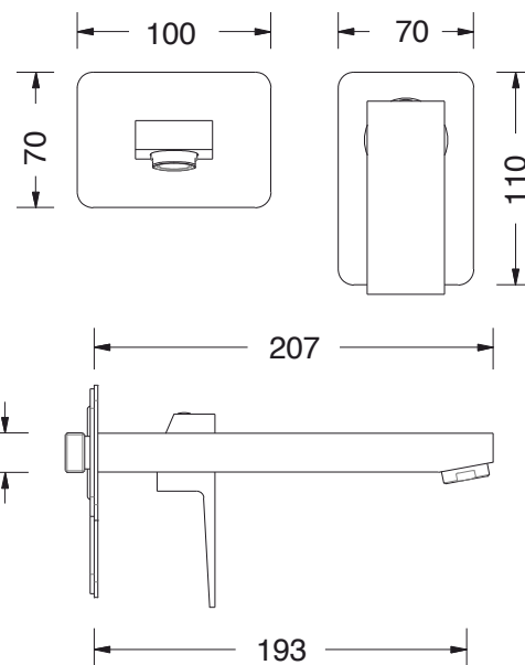
DISEGNO - DRAWING
