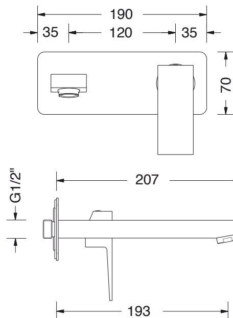
DISEGNO - DRAWING
