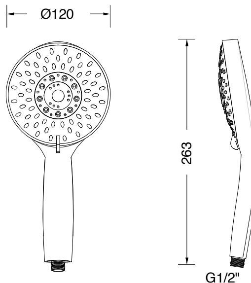
DISEGNO - DRAWING
