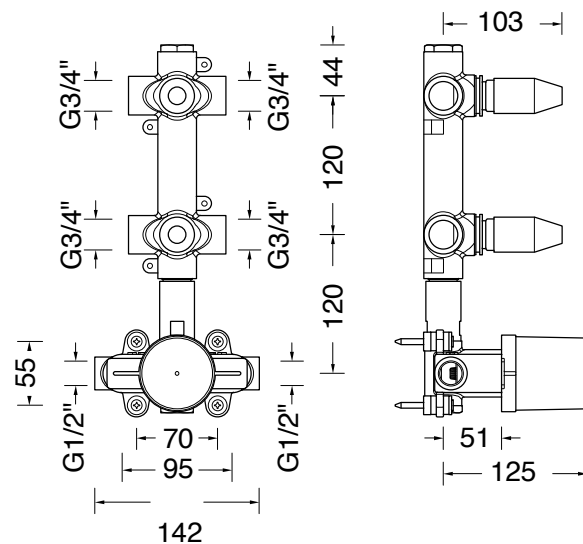
DISEGNO - DRAWING
