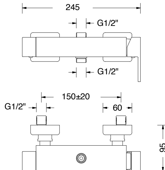
DISEGNO - DRAWING
