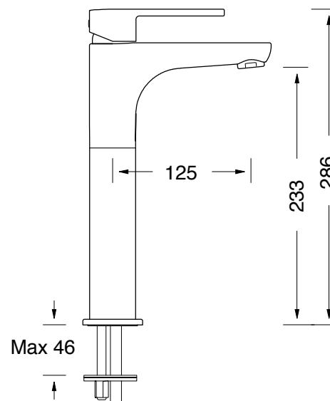
DISEGNO - DRAWING
